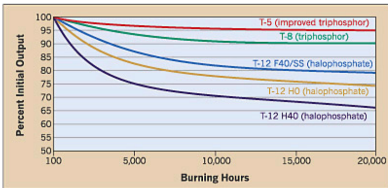
เปรียบเทียบการคงค่าความสว่างตามอายุการใช้งาน (Lumen maintenance) ของหลอดชนิดต่างๆ
